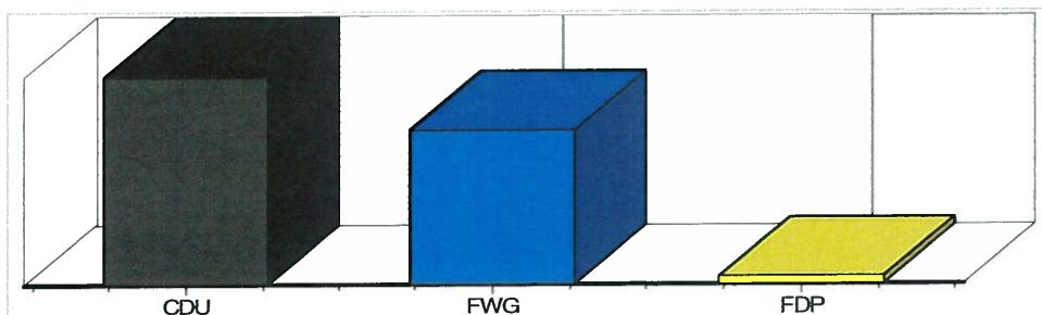
Abbildung 1: Stimmverteilung
