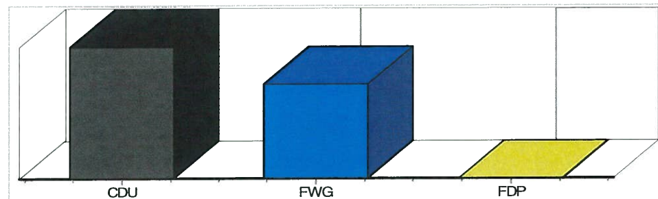
Abbildung 2: Sitzverteilung
